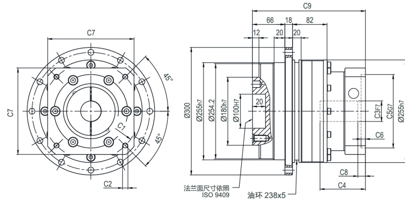
输入端/INPUT
