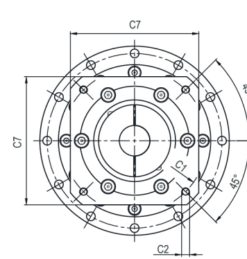
输入端/INPUT
