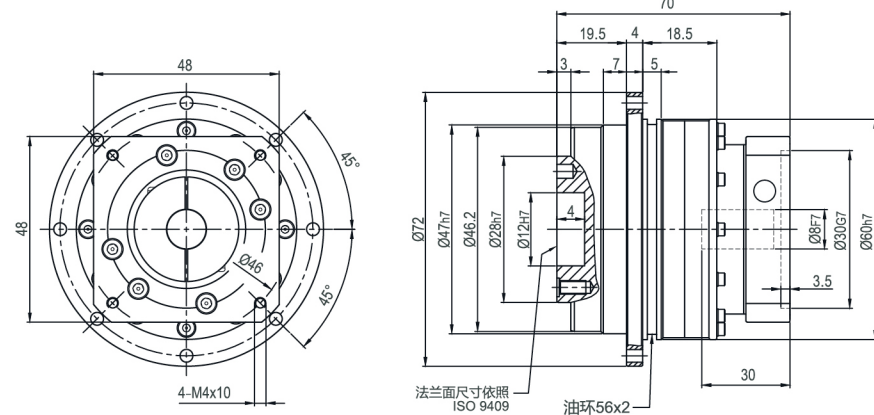
输入端/INPUT
