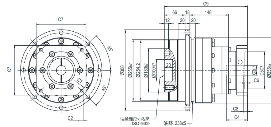
输入端/ INPUT
