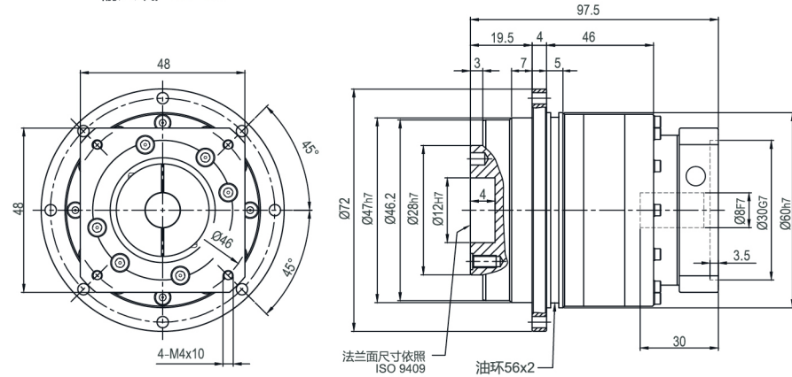
输入端/ INPUT
