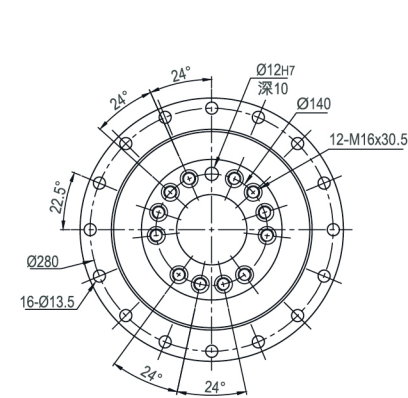
输出端/ OUTPUT
