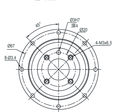
输出端 /OUTPUT
