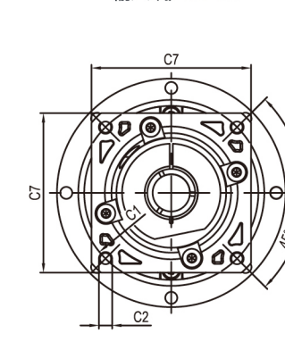
输入端/ INPUT
