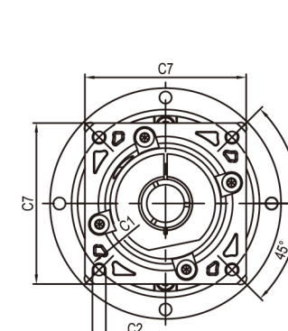
输入端/ INPUT
